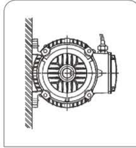
IM B6
