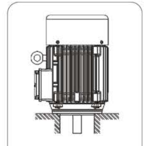
IM V18
