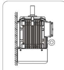
IM V6
