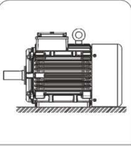
IM B3
