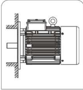
IM B5
