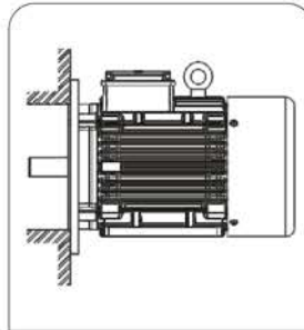
IM B35
